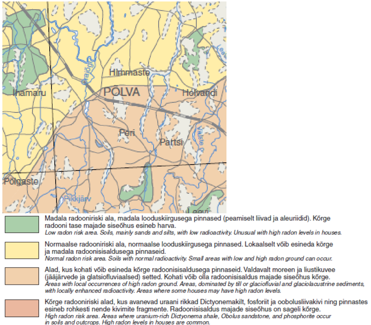
Joonis 6. Väljavõte Eesti radooniriski kaardist.
